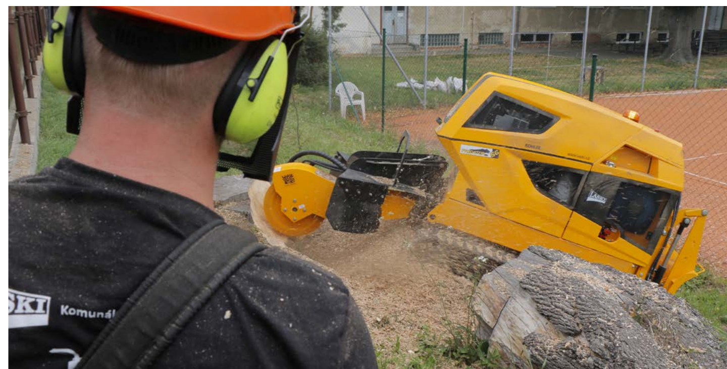
P 56 RX při testech / P 56 RX at field tests
